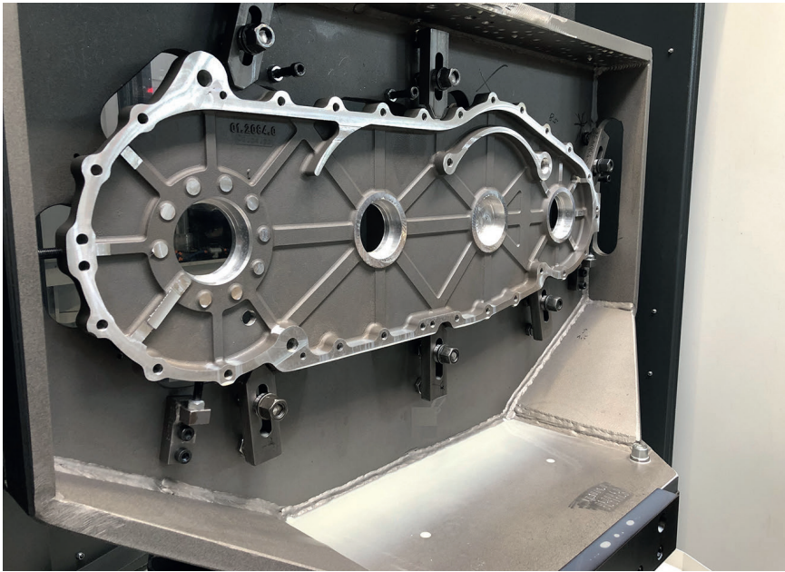
2 Eines von Tausenden Fertigungsteilen von Kordel – ein Getriebegehäuse aus Aluminium, bearbeitet mit Werkzeugen aus dem automatisierten Magazin © Kordel
